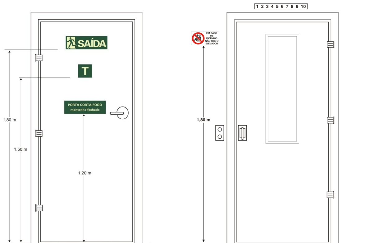
Figura C-3 - Sinalização de porta corta-fogo. Figura C-4 - Sinalização de elevadores (vista da escada).
