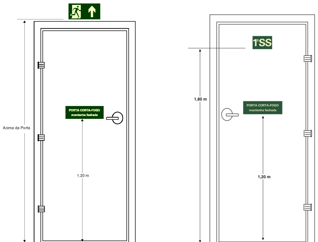
Figura C-1 - Sinalização de porta corta-fogo (vista da escada). Figura C-2 - Sinalização de porta corta-fogo (vista do hall).
